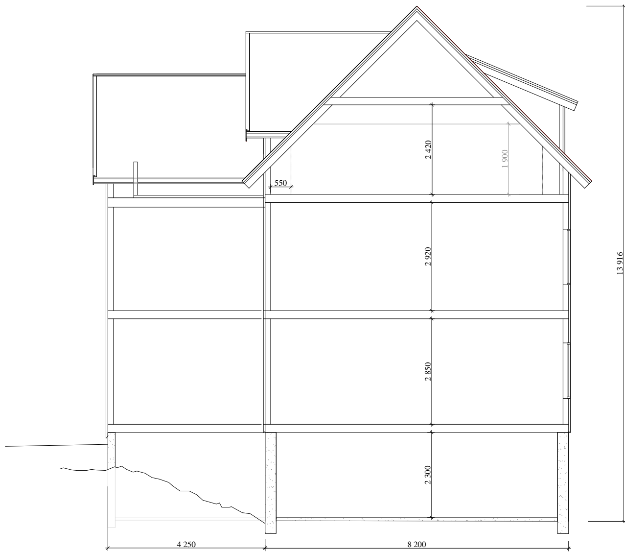
SNITT FASADE SØR
